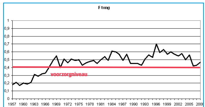
Figuur 1: Historische ontwikkeling visserijdruk Noordzeetong
